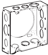
73171 1/2 & 3/4
